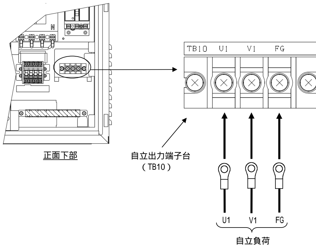
図 5-7 自立出力端子台接続図
