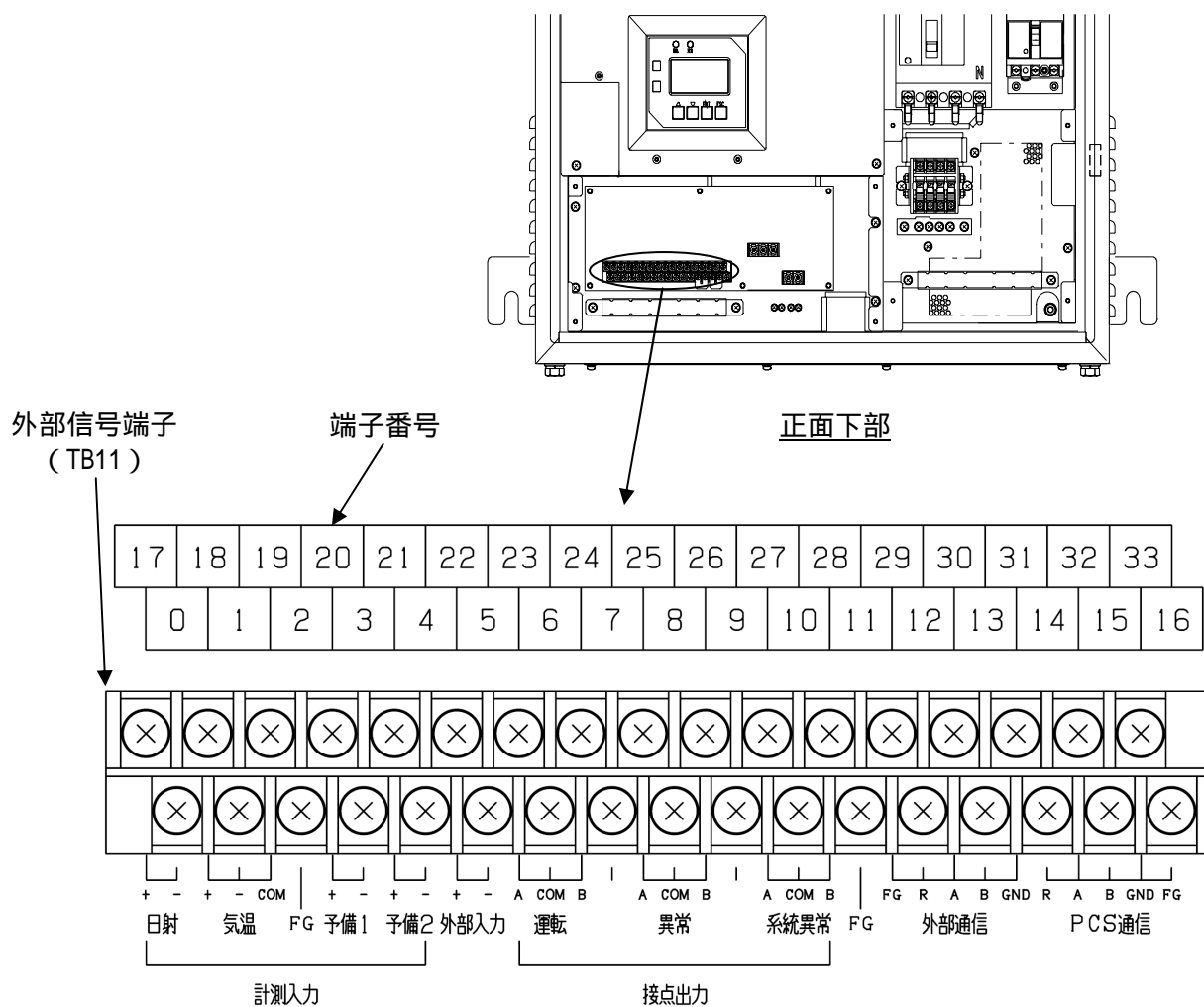
図 5-5 外部信号端子ピンアサイン
