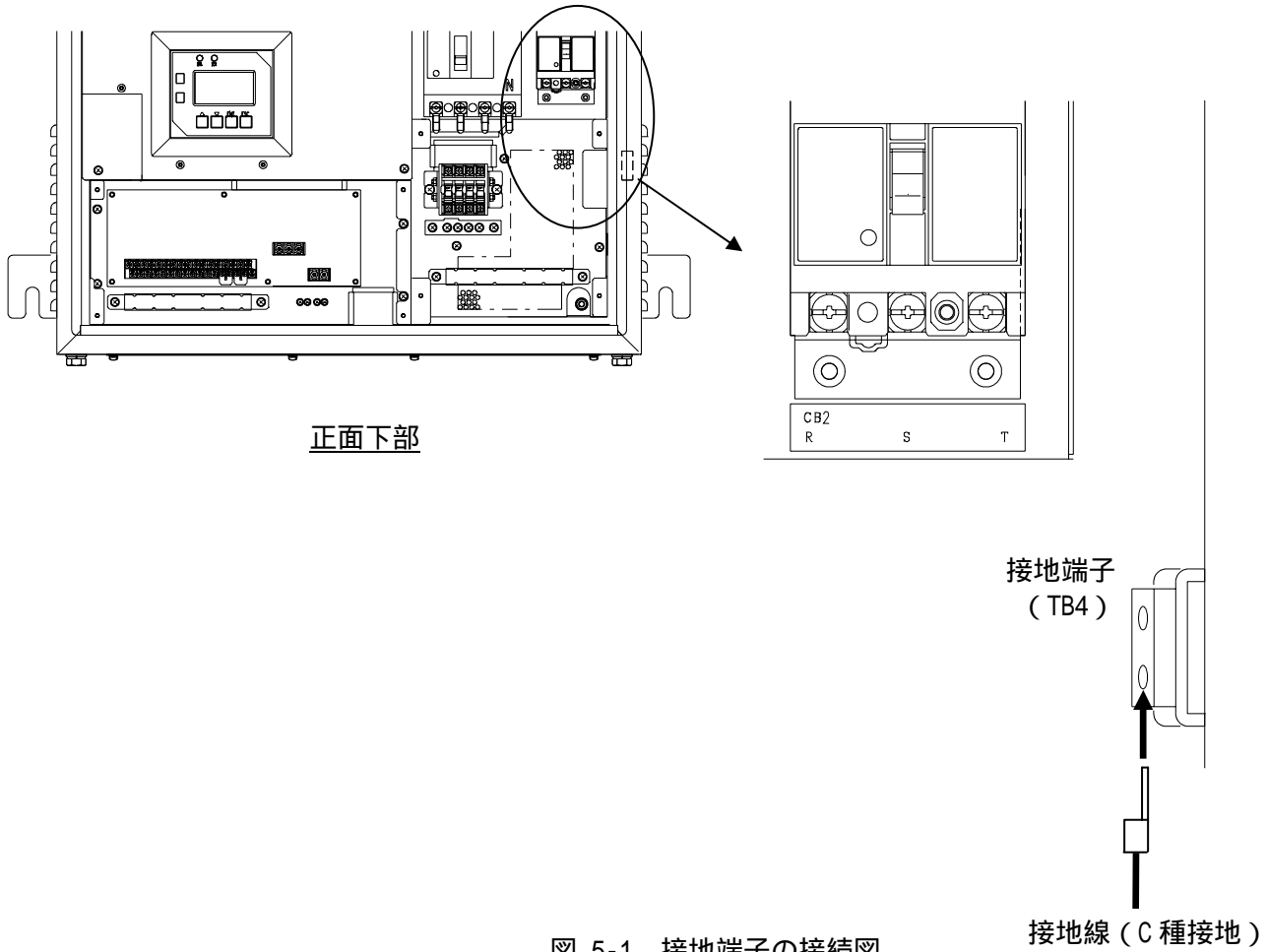
図 5-1 接地端子の接続図
