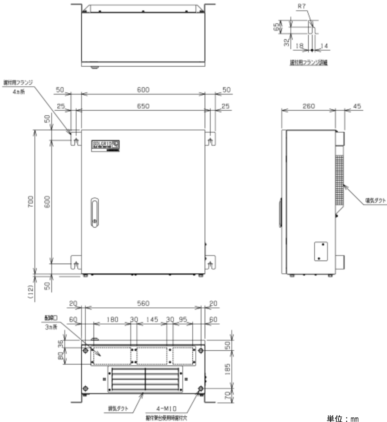
図 8-1 太陽光発電用パワーコンディショナ（標準品）の外形寸法図
