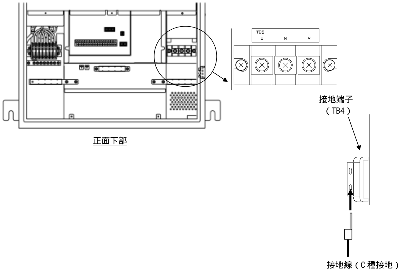
図 5-1 接地端子の接続図
