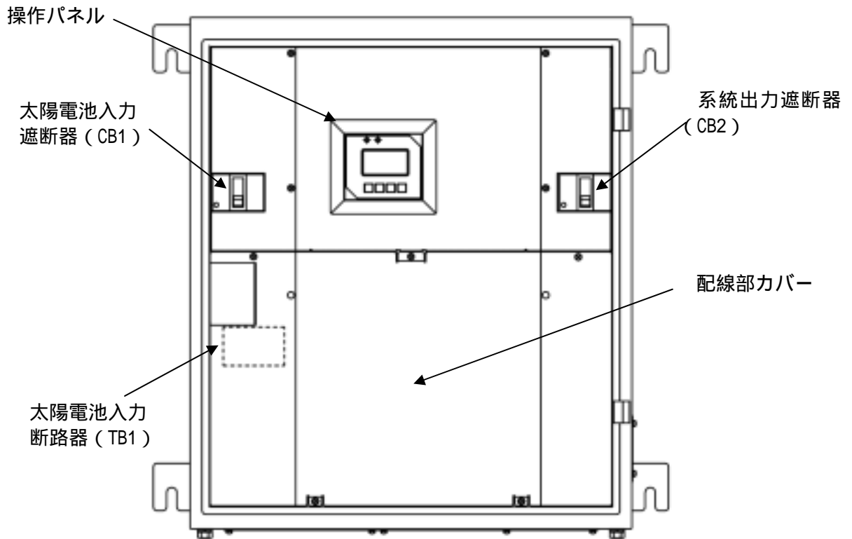
図 3-3 太陽光発電用パワーコンディショナの扉を開けた状態
