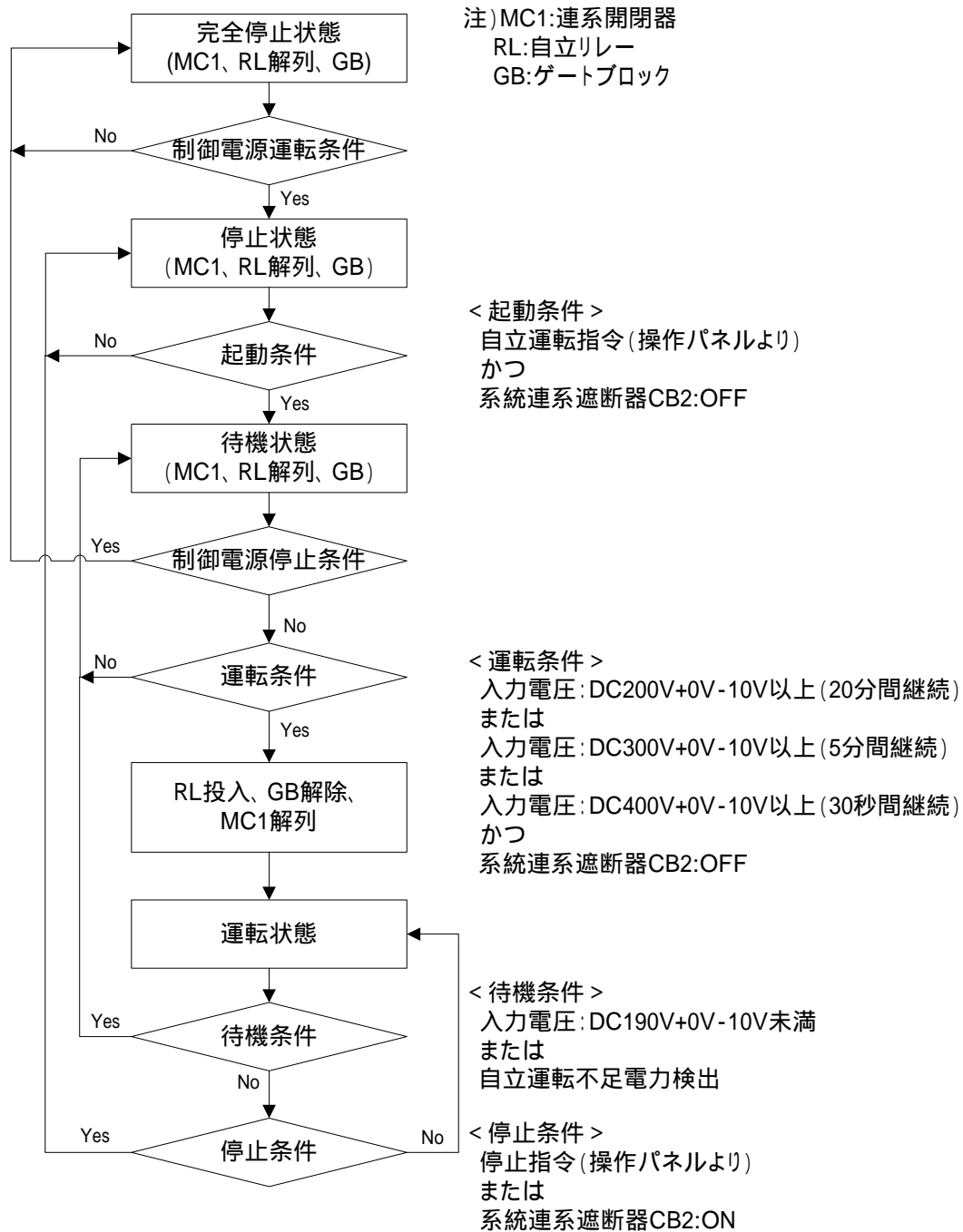
図 8-4 自動起動・停止フローチャート(自立運転)
