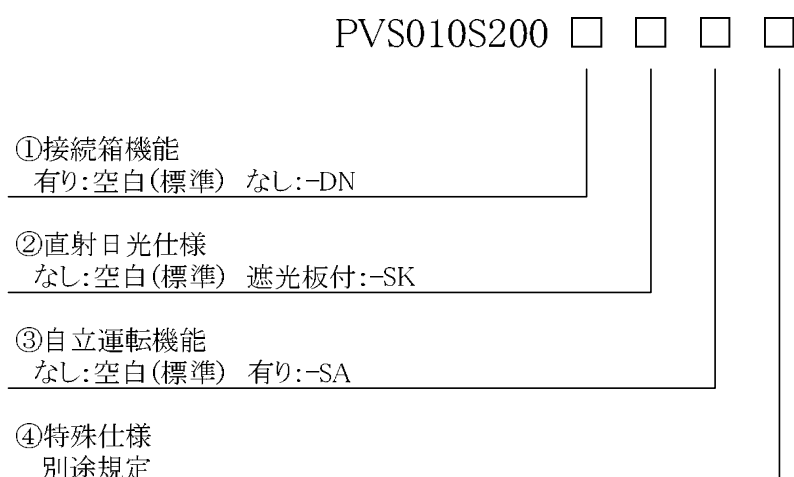
図 2-1 型名とオプション
