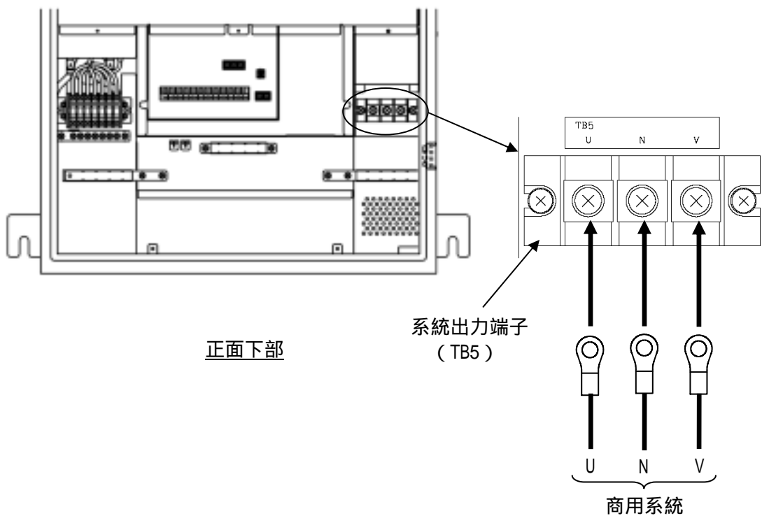
図 5-4 系統出力端子接続図
