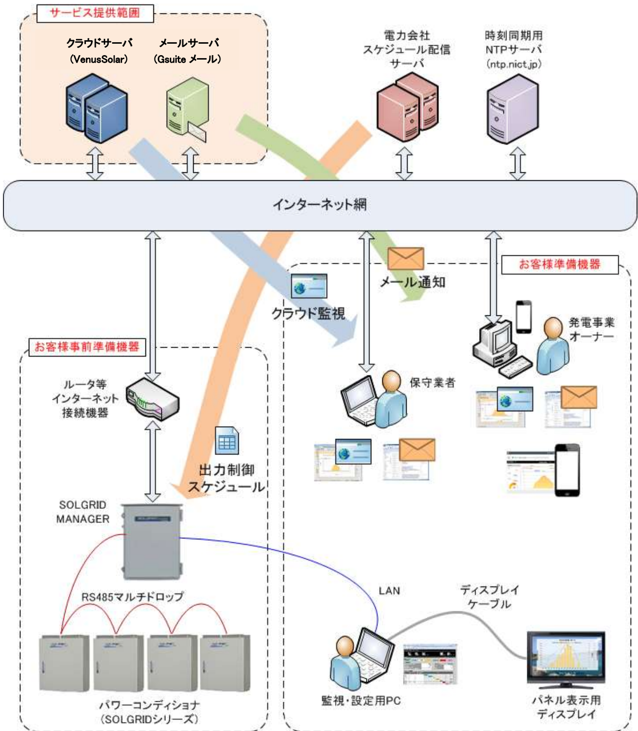
図2 LAN 接続方式(有線方式)の場合
