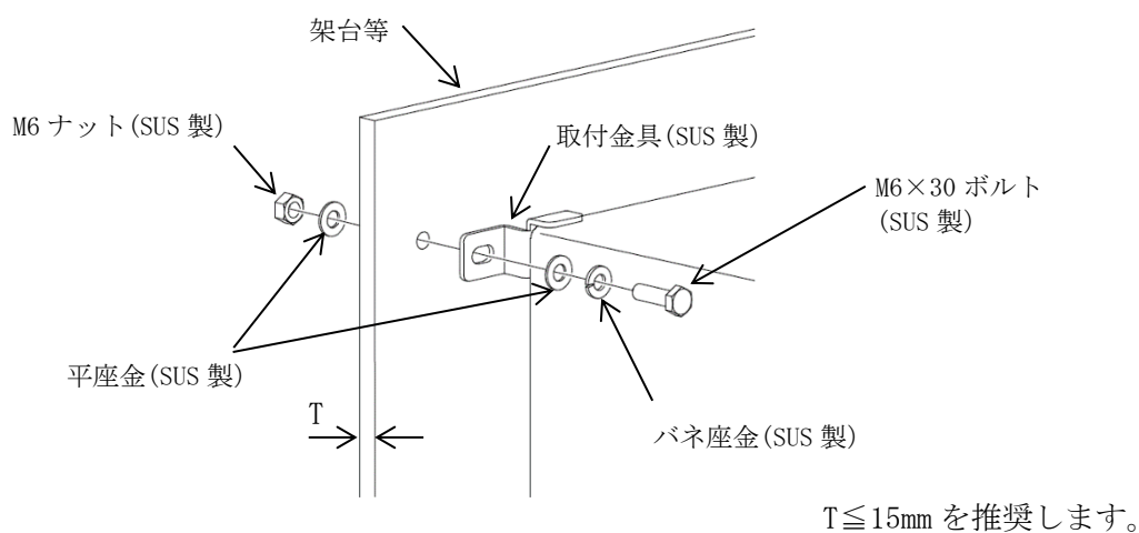
図 4.2-2 固定方法
