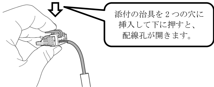
図 4.3-2 絶縁抵抗試験-2
