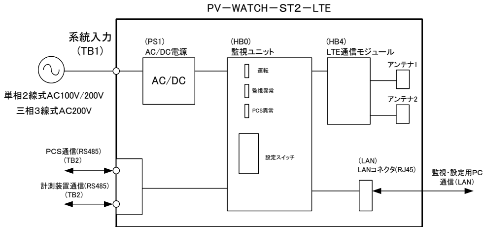
図 2.6-1 回路系統図(PV-WATCH-ST2-LTE)
