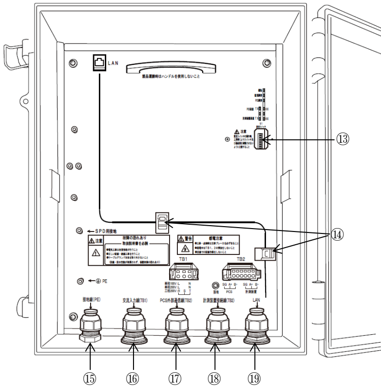
図 3.2-4 内部構成 (PV-WATCH-ST2-LAN) (中カバー脱却時)
