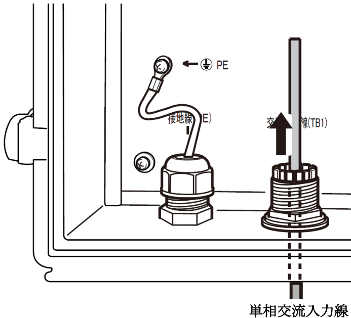
図 5.6-1 単相電源線の配線-1
