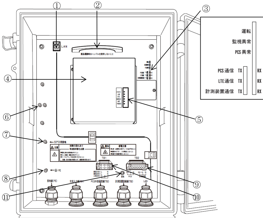
図 3.2-1 内部構成 (PV-WATCH-ST2-LTE) (中カバー装着時)
