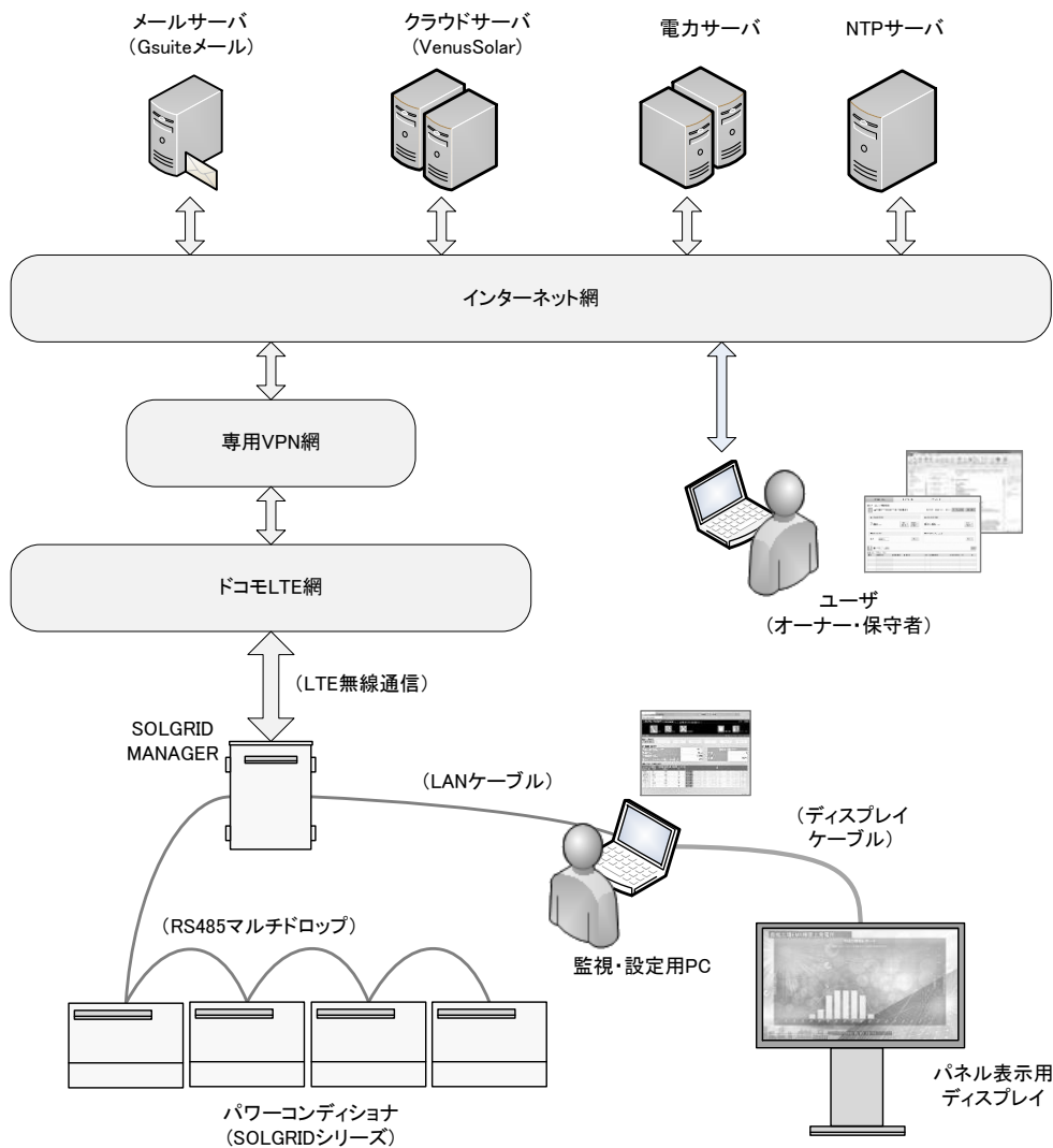
図 2.5-1 システム構成の例 (PV-WATCH-ST2-LTE)
