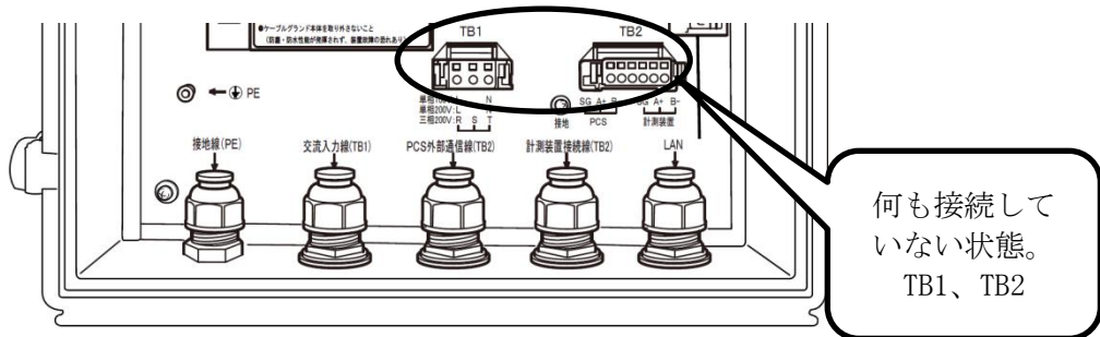
図 4.3-1 絶縁抵抗試験-1
