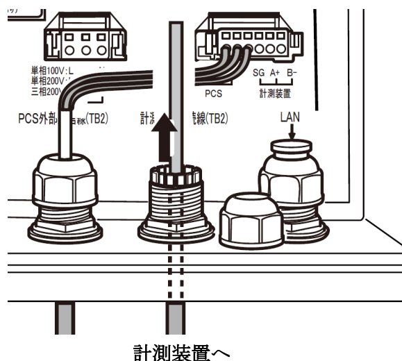
図 5.4-2 計測装置との RS-485 接続-2
