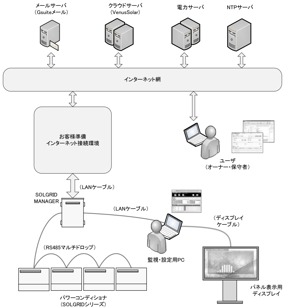
図 2.5-2 システム構成の例(PV-WATCH-ST2-LAN)
