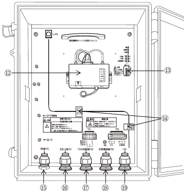
図 3.2-2 内部構成 (PV-WATCH-ST2-LTE) (中カバー脱却時)
