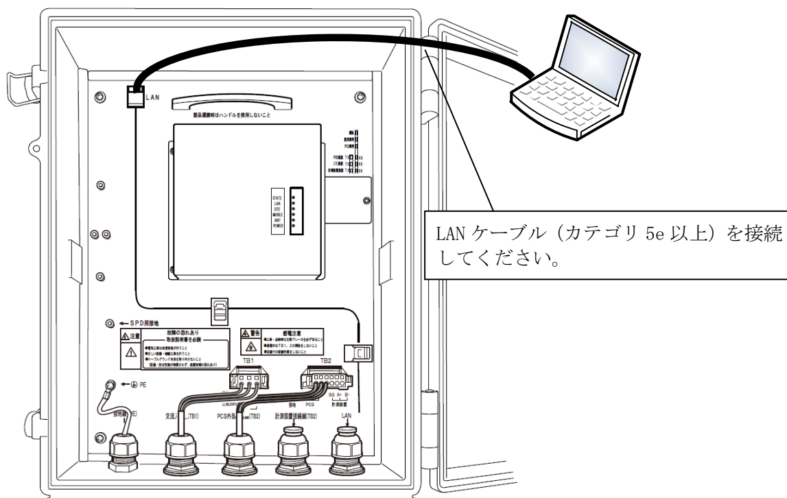
図 5.9-1 PC との LAN 接続-1
