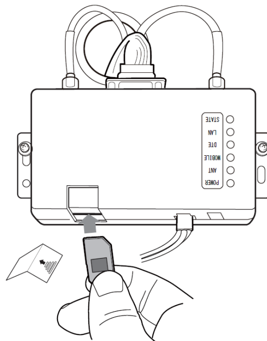
図 5.8-4 SIMカードの挿入-4
