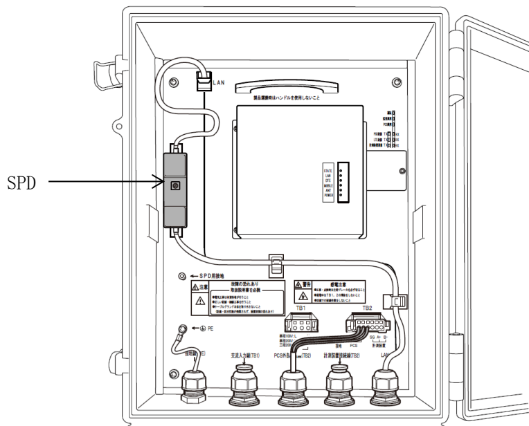
図 5.5-2 PC との LAN 常時接続 (PV-WATCH-ST2-LTE)-2
