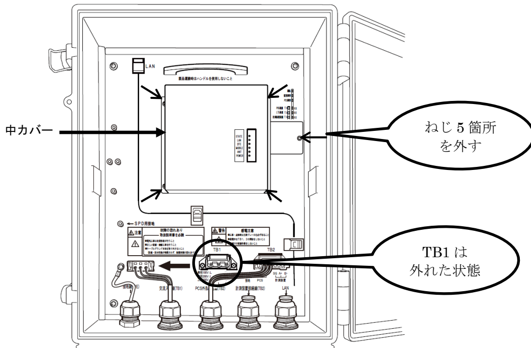
図 5.8-1 SIM カードの挿入-1
