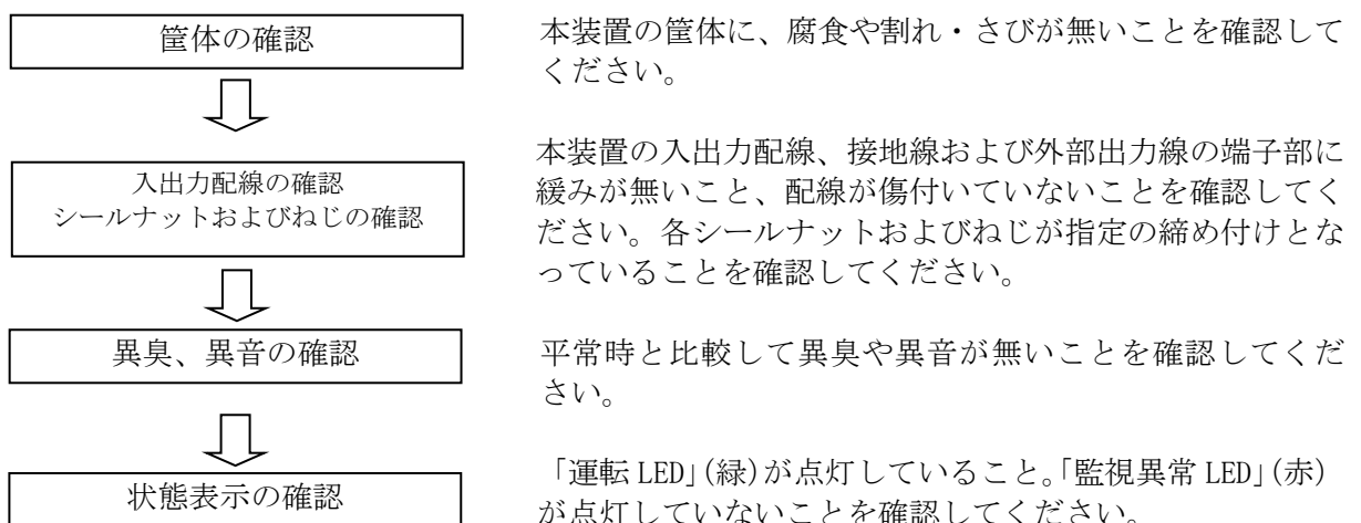
図 7.1-1 定期点検
