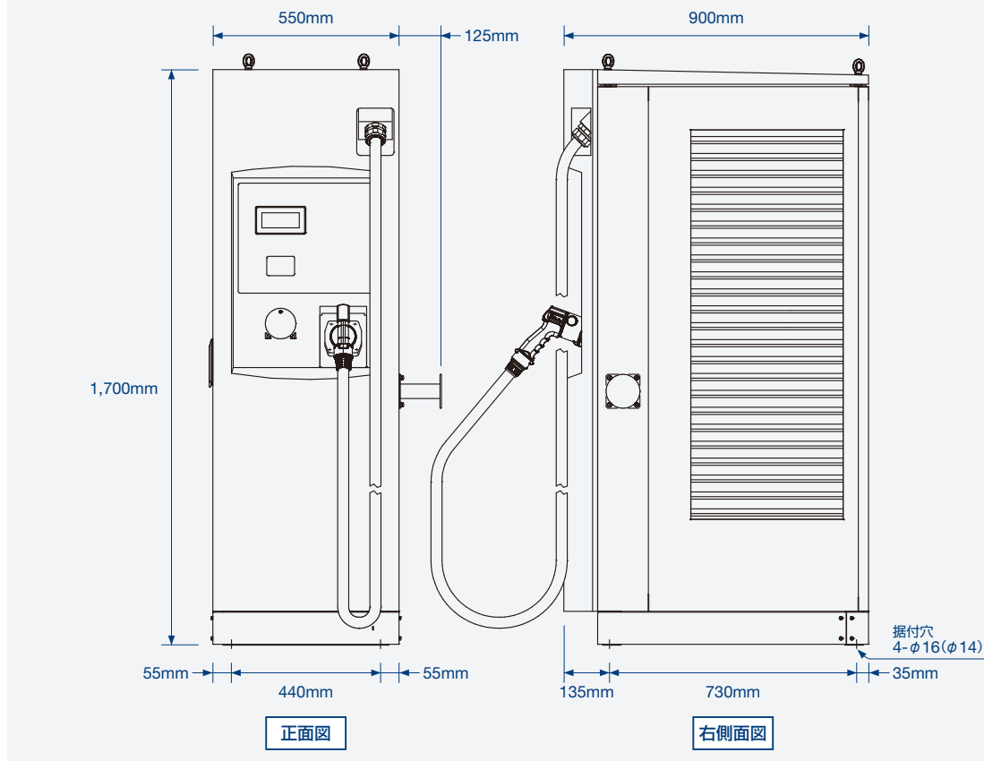
外形図 SDQC-301
