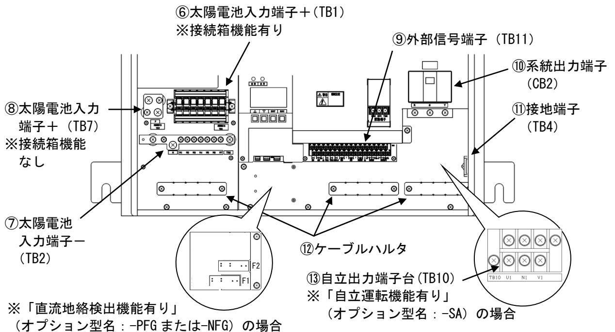
図 7-4 太陽光発電用パワーコンディショナの配線部カバーを外した状態 (標準品)
