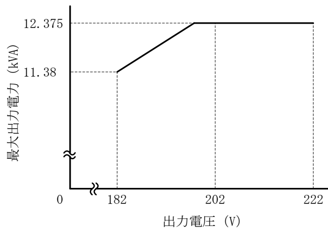
図 12-7 出力電圧制限特性
