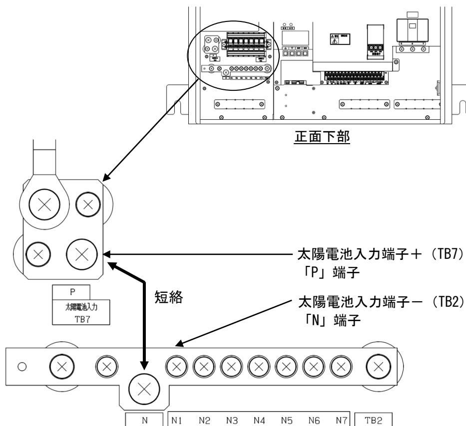
図 8-6 絶縁抵抗試験 太陽電池入力端子 接続箱機能なし
