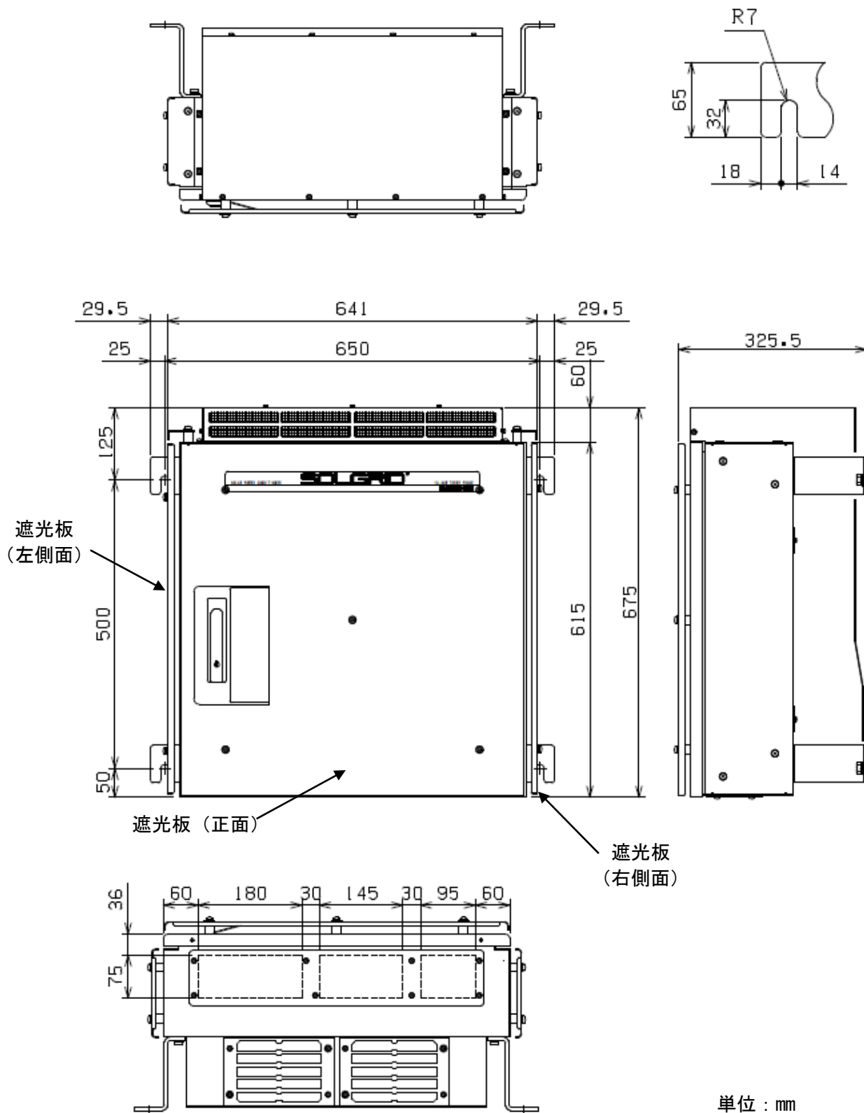
図 12-2 太陽光発電用パワーコンディショナ (オプション型名 : -SK) の外形寸法図
