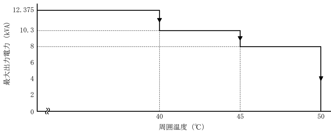
図 12-5 温度制限特性
