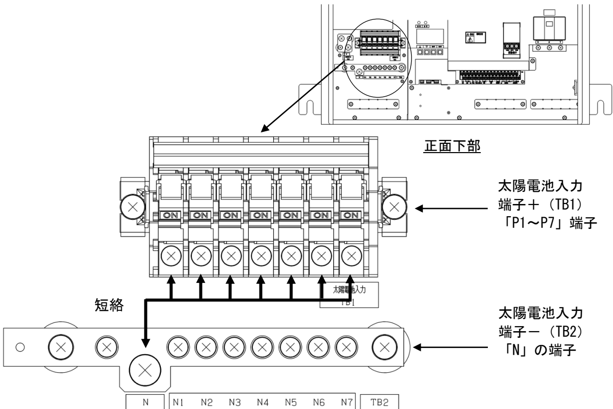
図 8-5 絶縁抵抗試験 太陽電池入力端子 接続箱機能有り
