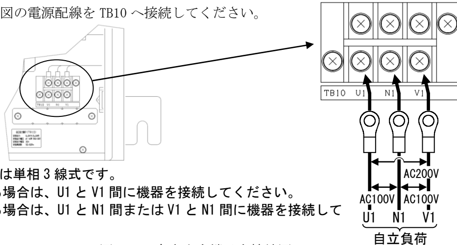
図 9-9 自立出力端子台接続図
