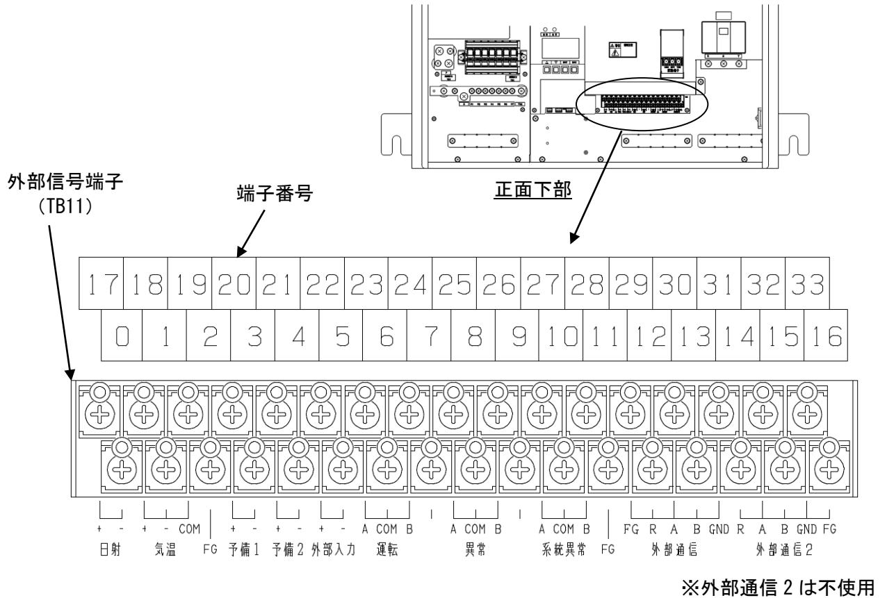
図 9-8 外部信号端子ピンアサイン
