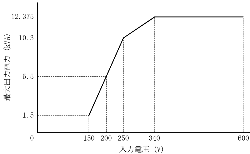
図 12-6 入力電圧制限特性
