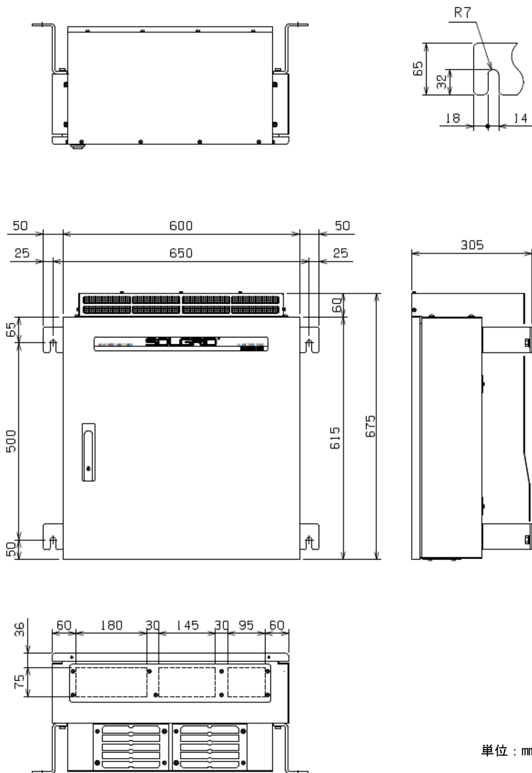
図 12-1 太陽光発電用パワーコンディショナ (標準品) の外形寸法図
