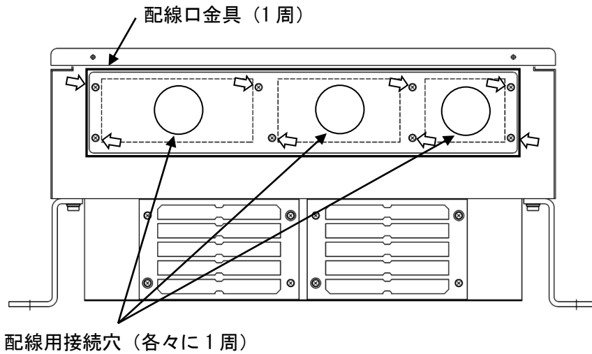
図 9-2 配線口金具の防水処理
