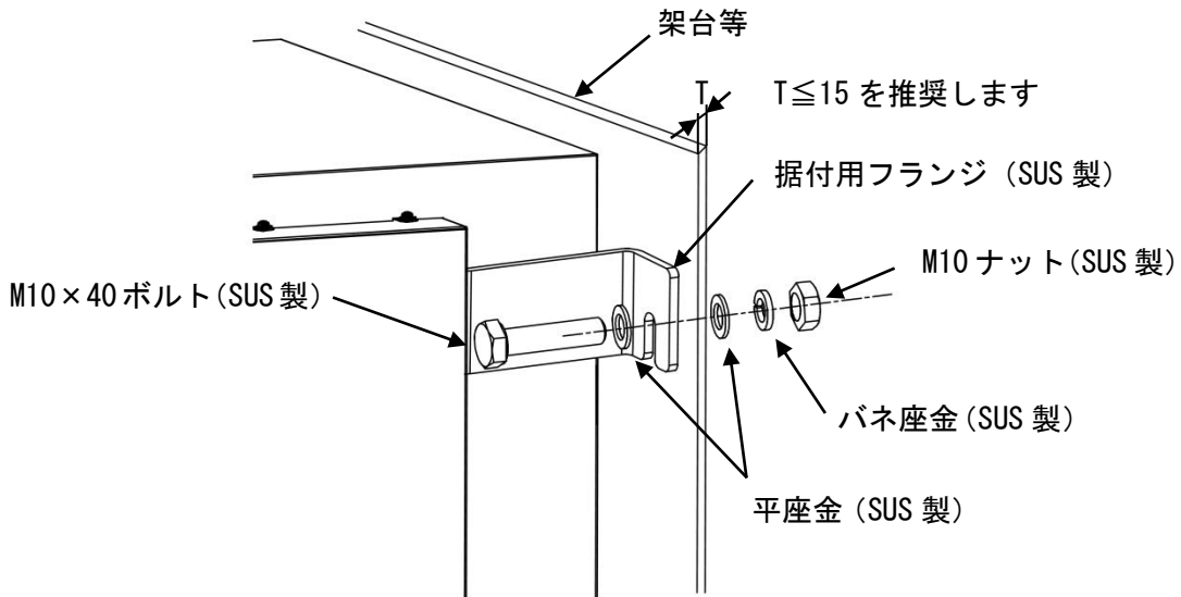
図 8-3 据付用フランジの固定方法
