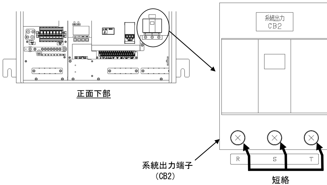
図 8-7 絶縁抵抗試験 系統出力端子
