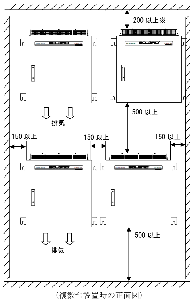
図 8-1 設置条件
