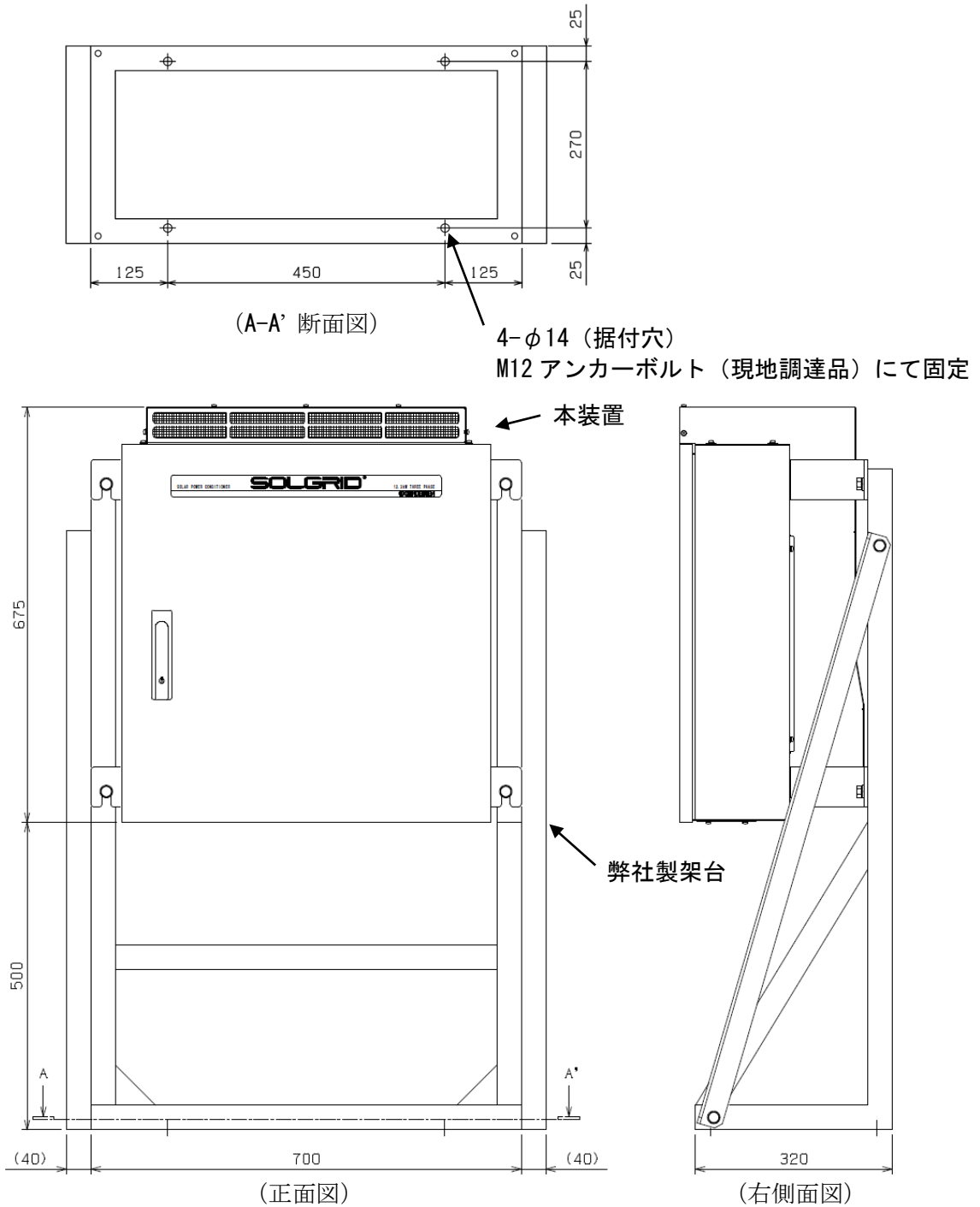
図 8-4 据置の設置方法
